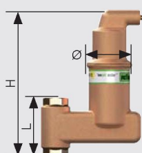
'exair solar' • κάθετο A 22 SV - A 1 SV
