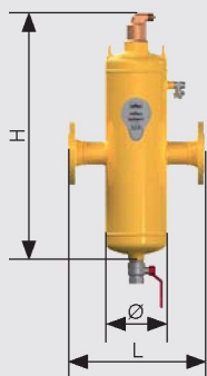
'extwin' TW 50 - 300
