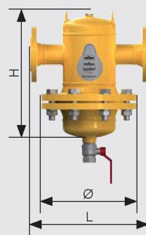
'exdirt' με φλάντζα επιθεώρησης D 50 R - 300 R
