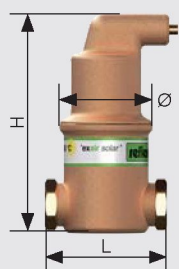
'exair solar' A 22 S - A 1 1/2 S
