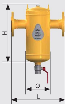
'exdirt' D 50 - 300
