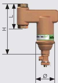
'exdirt' • κάθετο D 22 V - 1
